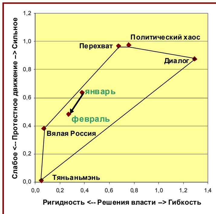
Рисунок 3. Диаграмма взаимного расположения сценариев в политическом пространстве сегодняшней России. Точки, помеченные надписями «январь» и «февраль», характеризуют политическое положение в стране на соответствующие моменты времени по результатам прогнозирования
